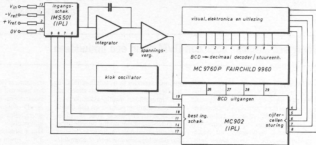
Fig. 2. Standaard blok-schema van de DPM, werkend volgens het principe van de opeenvolgende spannings- en ontladingsimpulsen integratie (dual slope). De MC902 maakt een sterk vereenvoudigde opzet mogelijk.
