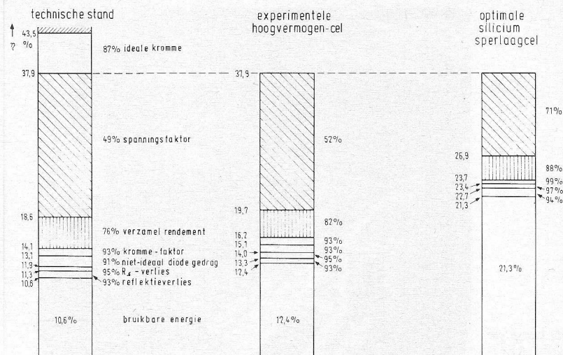
Fig. 13 Ontwikkelingsmogelijkheden voor zonnecellen.
