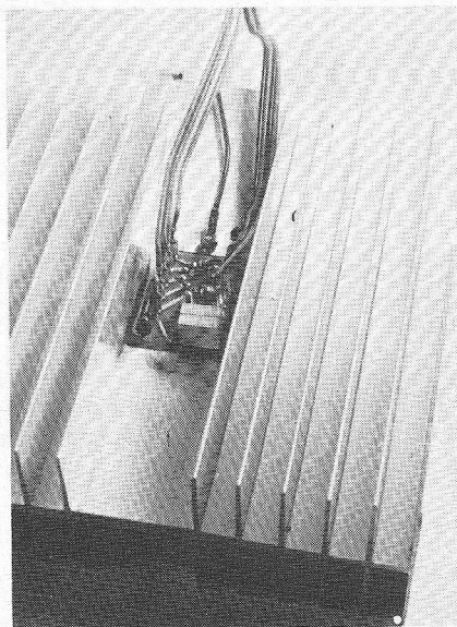
Afb. 2. Montage van de spanningregelaar op het printje in de koelplaat.
