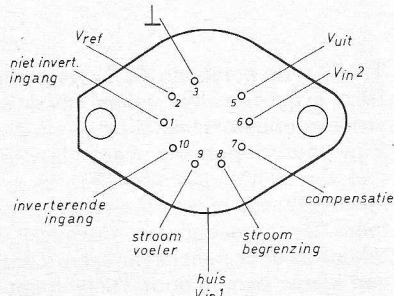
Fig. 6. Aansluitgegevens
