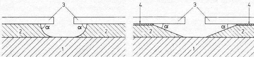
Fig. 1. a Conventionele etsmethode; fig. 1b nieuwe etsmethode.
