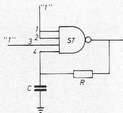
Fig. 10d. Met een hoog ingangsignaal geeft de uitgang impulsen af.
