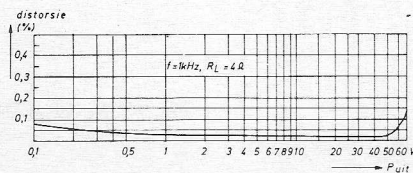
Fig. 15. Karakteristiek van de schakeling uit fig. 14.
