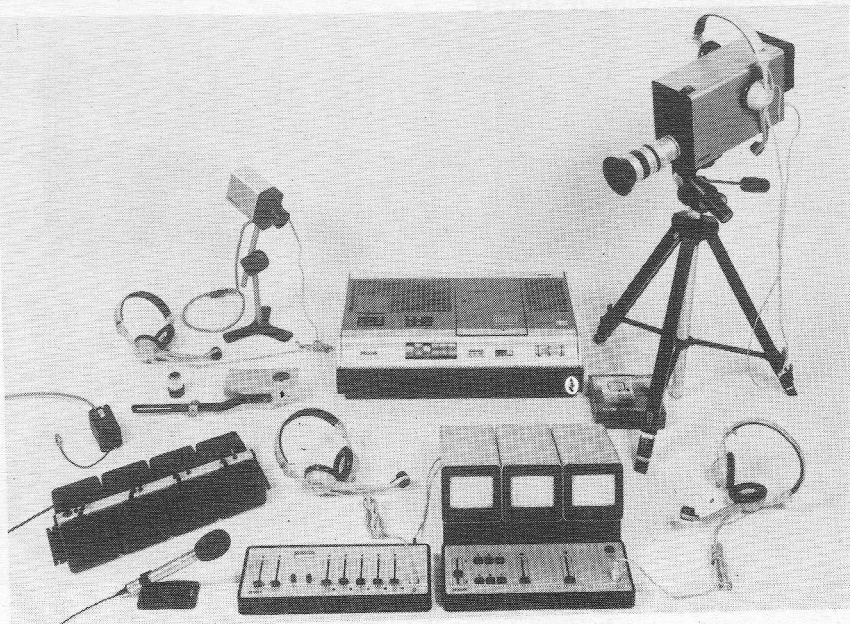
Afb. 1. Complete 2-camera studio van Philips.
