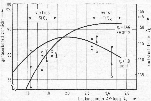
Fig. 14 Verbetering van de lichtabsorptie door aangepaste brekingsindex van de anti-reflexlaag.
