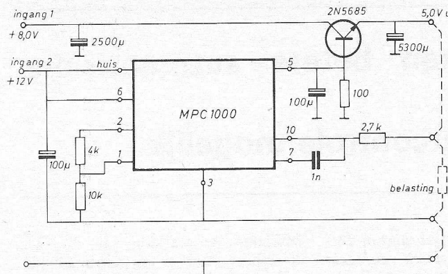
Fig. 4. Spanning-regelaar 5 V bij een stroom van max. 50 A met sense aansluitingen.
