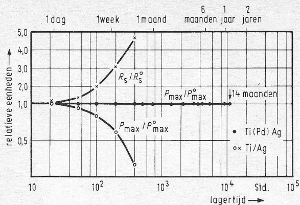
Fig. 15 Daling van het elektrische uitgangsvermogen P_{\max} als functie van de tijdsduur van een lagerbehandeling met vocht ( T = 90^\circ\text{C} ).
