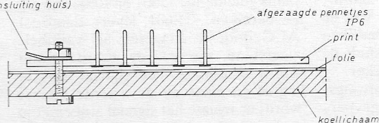
Fig. 5. Montage van het printje boven de koelplaat, waarop alleen de condensatoren zijn aangebracht volgens fig. 2.
