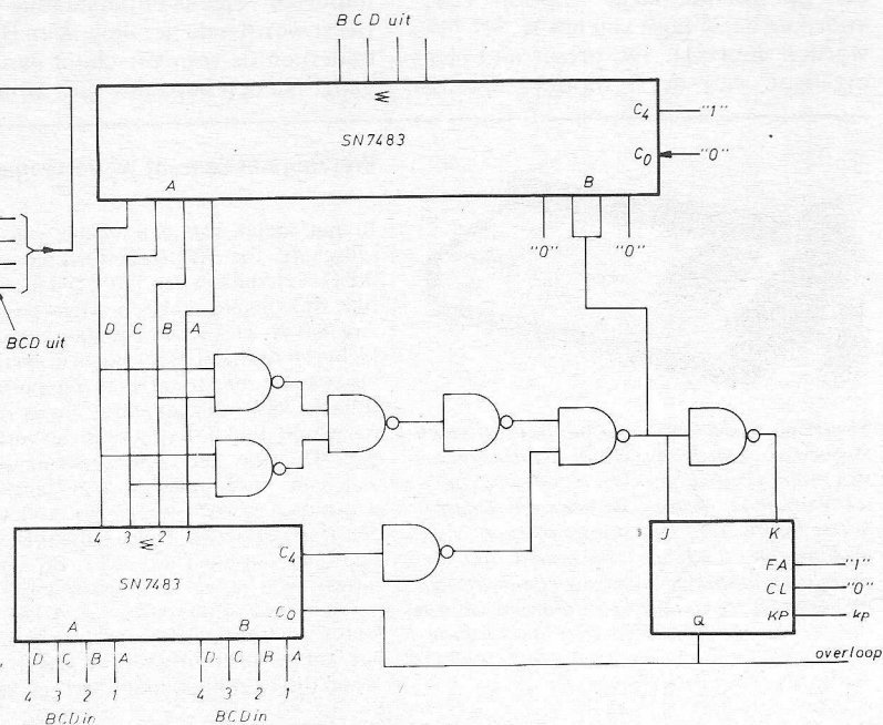
Fig. 2. Optelschakeling.
