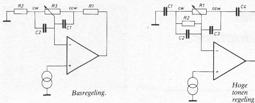
Fig. 2. Lage en hoge tonen regelcircuits met karakteristieken als van de schakeling in fig. 1.
