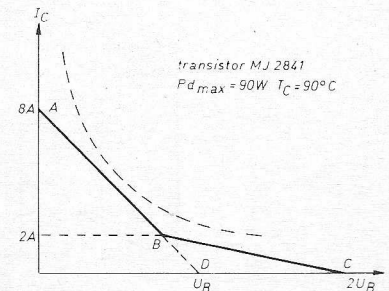
Fig. 15. Karakteristiek van de schakeling uit fig. 14.
