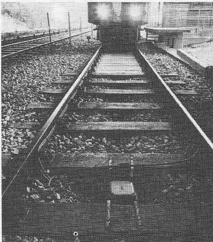
Afb. 1. Lijngeleider van de elektronische informatieverbinding.
