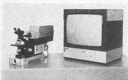
Afb. 4 Kleuren telemicroscoop CSW 3 van Schlumberger.
