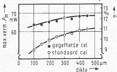
Fig. 11 Invloed van het getter-proces op vermogen en rendement van een zonnecel.
