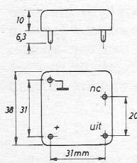
Fig. 1. Afmetingen van de oscillator.
