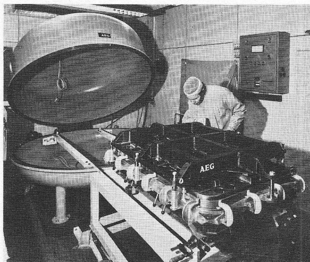
Afb. 4. In de vacuümkamer wordt in één arbeidsgang de complete layout van het zonnepaneel op de structuur geplakt. (foto's: AEG-Telefunken).
