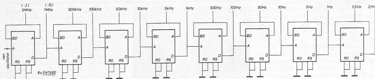
Fig. 3. Frequentiedeler.
