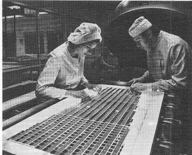
Afb. 3. Een paneel met zonnecellen wordt klaar gemaakt voor plaatsing in de, op de achtergrond „zichtbare”, vacuümkamer.
