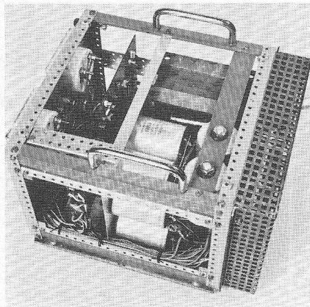
Afb. 2. Interieur van de afgemonteerde voeding.
