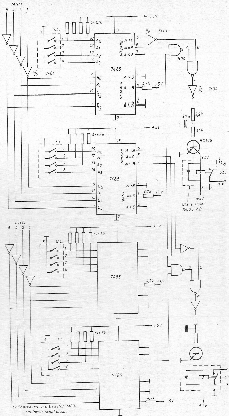
Fig. 2. Principe van de grenswaarde schakeling.
