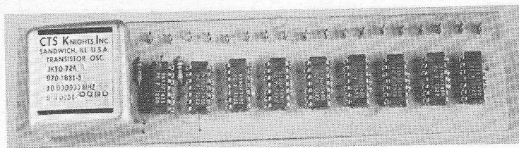
Afb. 1. Printje van de tijdbasis. Enkele componenten bevinden zich onder de oscillator. Inmiddels is de oscillator verbeterd en aangepast op TLL-niveau. Voor een fan-out van 10 blijft de buffertrap noodzakelijk.
